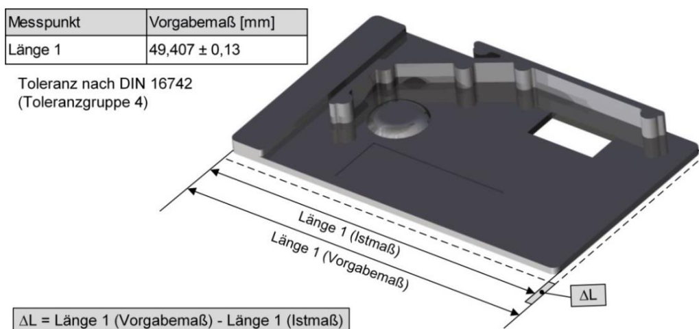
Bild 2: Das Testprodukt der Phoenix Contact GmbH & Co. KG. (Bildquelle: Phoenix Contact)
